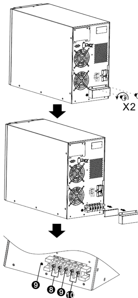
端子视图
